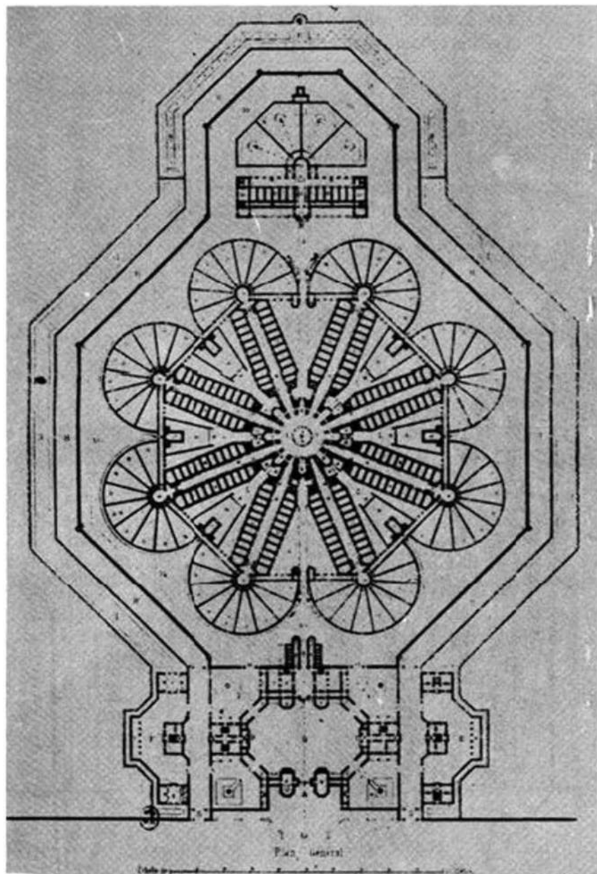
A. Blouet, 585 mahkûmluk hücreli hapisane projesi, 1843.
